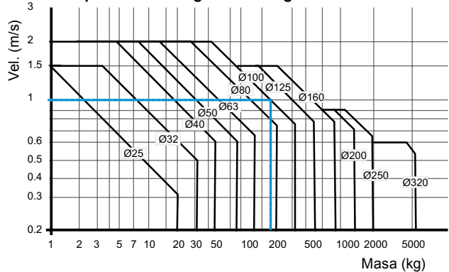
Gráfico Capacidad de Carga de amortiguación
